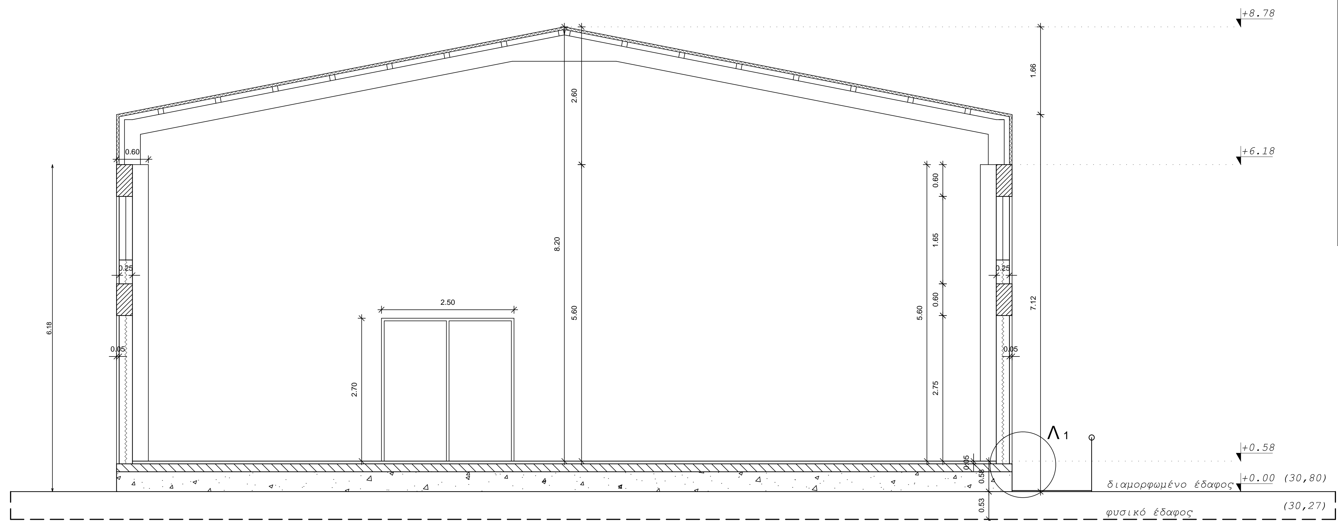
ΤΟΜΗ Α-Α
