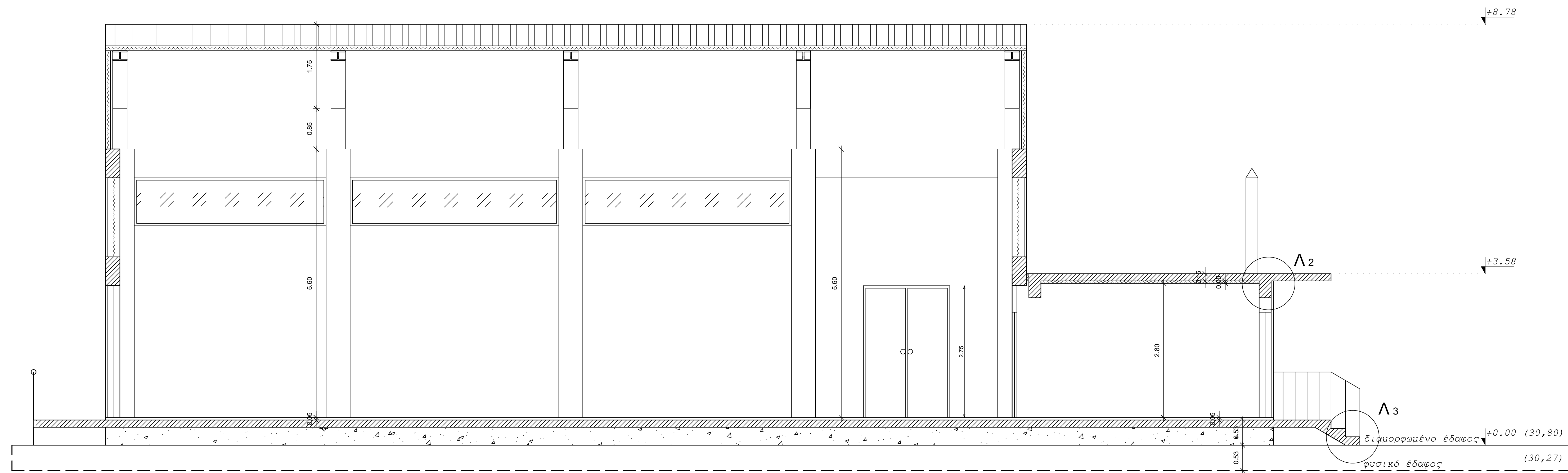
ΤΟΜΗ Β-Β
